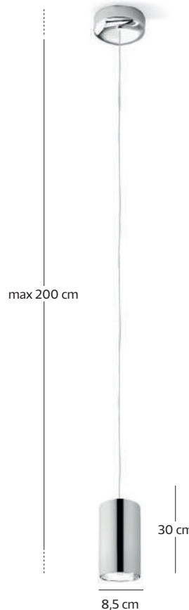
art. Planet S 30 1x GU. 10 Max 30 W
