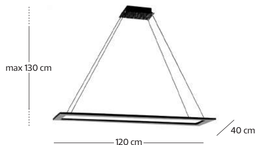
art. KLAQ S 120 telaio altezza regolabile / frame with adjustable height max 12 cablaggi CP 200 / max 12 cables CP 200
