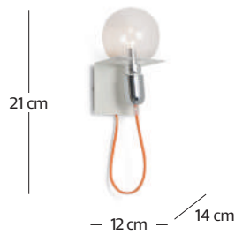
art. Bolle BLL A50 1 x max 28 W E27
