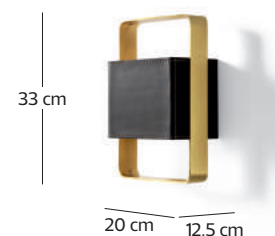
art. Contessa A20 2 x max 53 W E27
