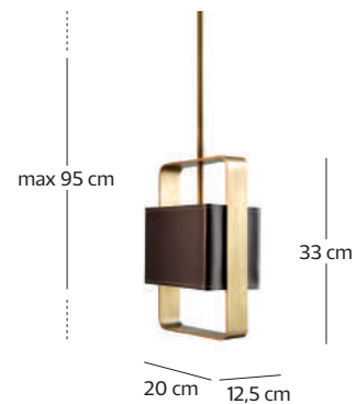
art. Contessa S20 1 x max 53 W E27
